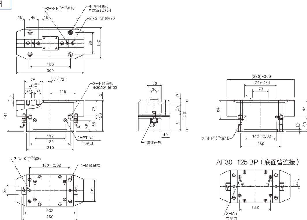
外形尺寸图
