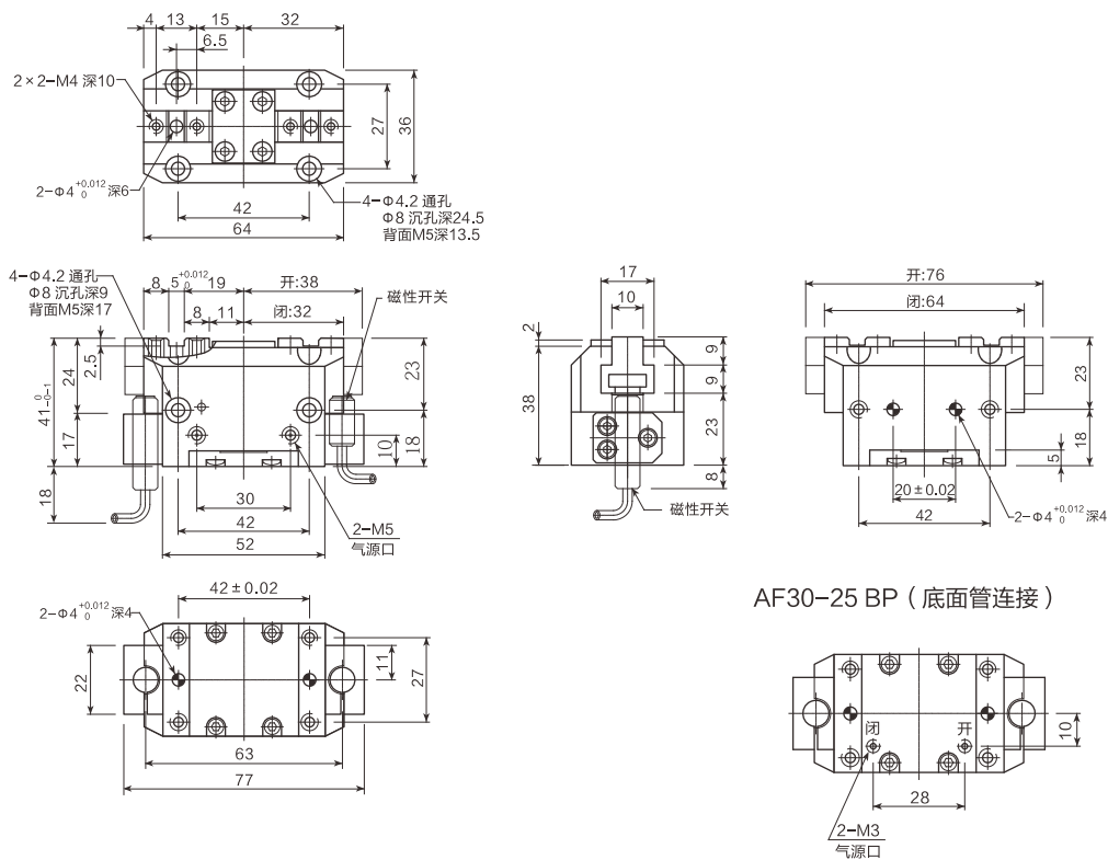
外形尺寸图
