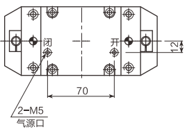
AF30-63 BP (底面管连接)
