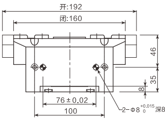
AF30-63 BP (底面管连接)
