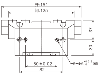
AF30-50 BP (底面管连接)
