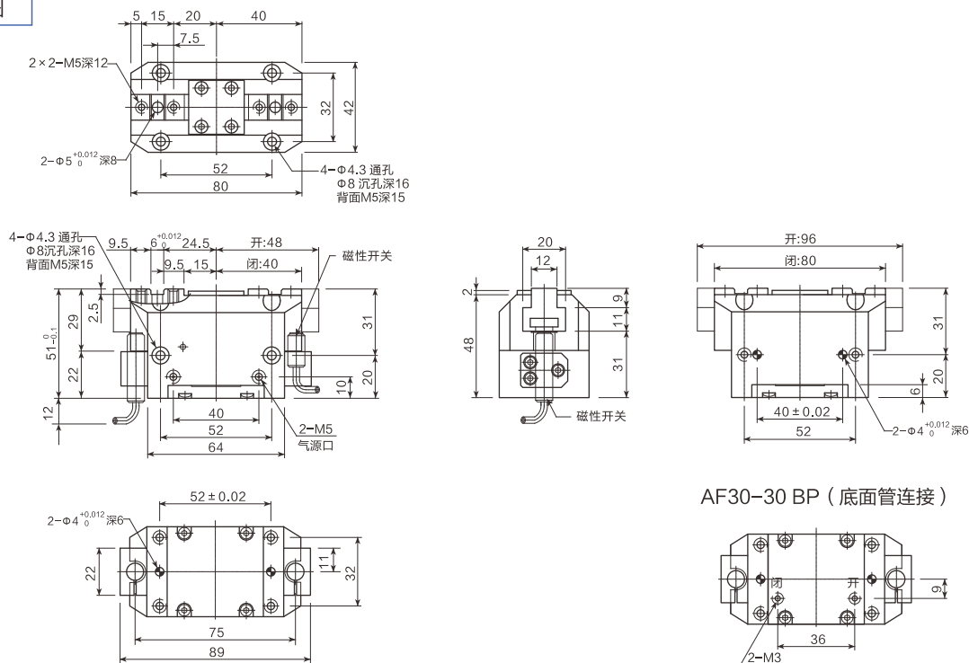
外形尺寸图
