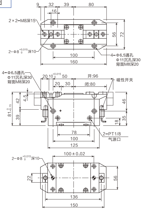
外形尺寸图
