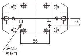
AF30-50 BP (底面管连接)
