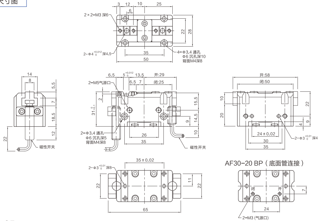
外形尺寸图
