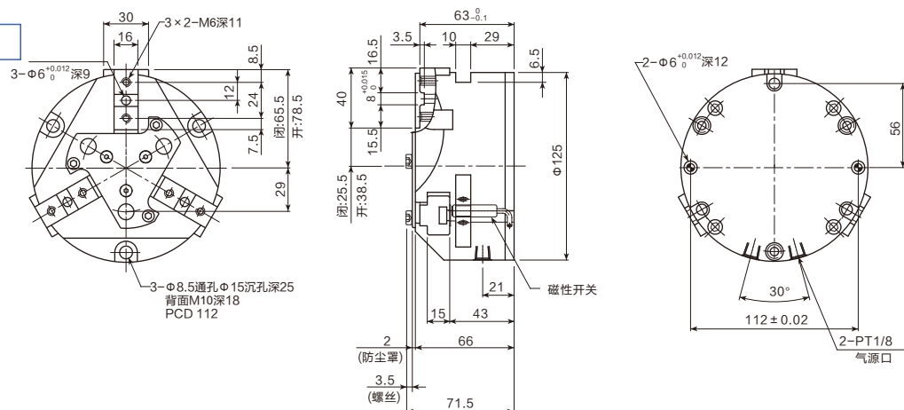
外形尺寸图
