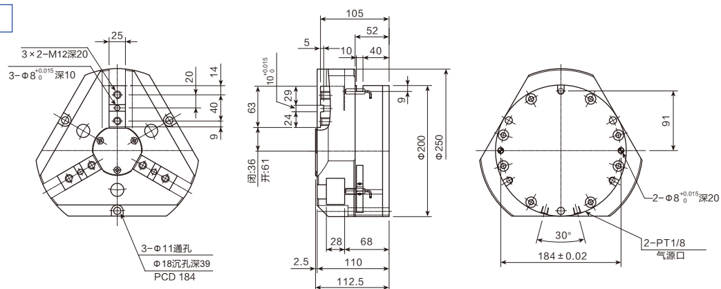
外形尺寸图
