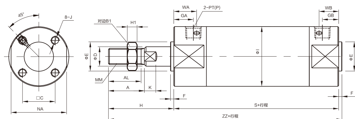
DHR2P尺寸图
