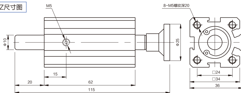
DHR2H25N15Z尺寸图
