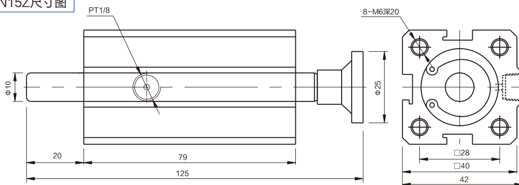
DHR2H25N15Z尺寸图
